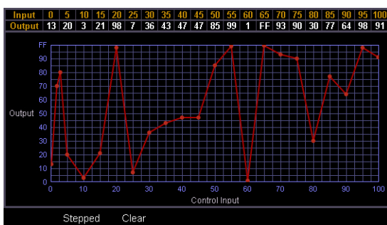
Interpolierte Kennlinie
