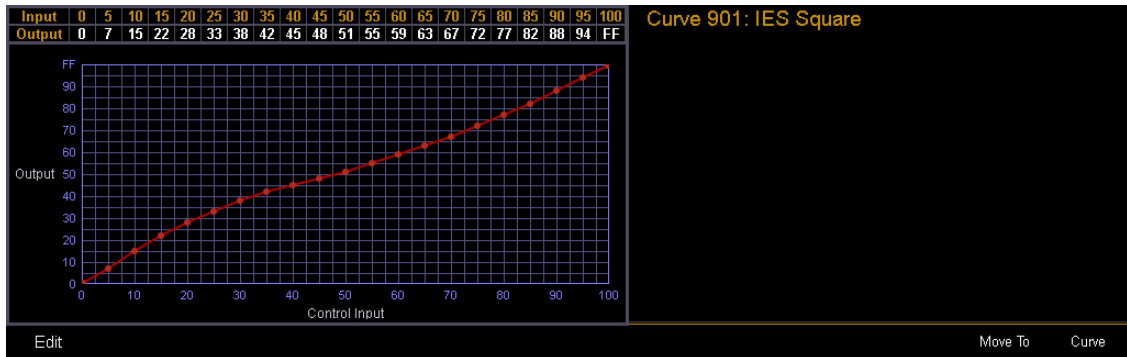
Vorprogrammierte Kennlinie
